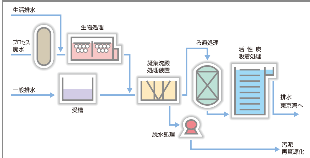
排水処理装置概略フロー図
