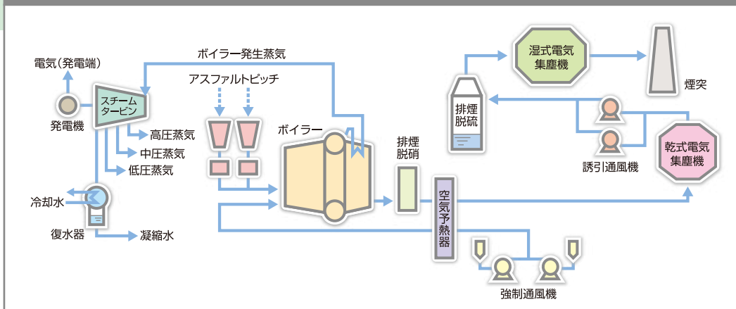
アスファルトピッチ焚きボイラー・タービン発電設備概略フロー図
