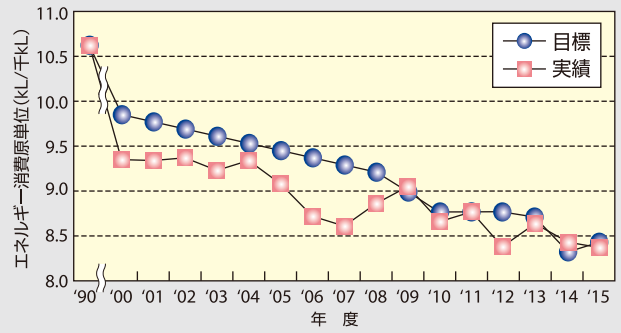
袖ヶ浦製油所エネルギー消費原単位推移
