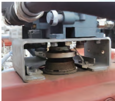
バルブ診断システムの導入 (弁開度の偏差で不具合を事前に検知可能)
