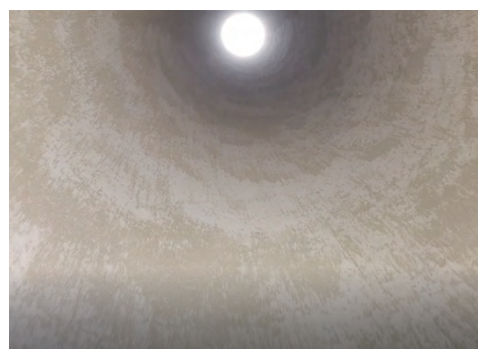
ドローンで撮影した煙突内部 (ライニングの健全性確認)
